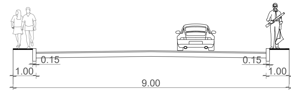
CALLE PRINCIPAL seccion transversal ESC: S/N
